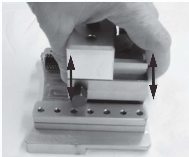
Figure 2-2. Ensuite, tentez d'incliner le charriot de l'avant vers l'arrière et de bas en haut. Cela peut s'avérer plus facile avec un outil installé sur le porte-outils, pour faire effet de levier.
