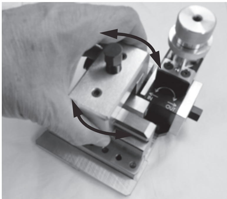
Figure 2-1. Une fois le plateau installé sur un établi, maintenez le charriot-outils et essayez de le faire bouger d'un côté à l'autre, entre les rails.
