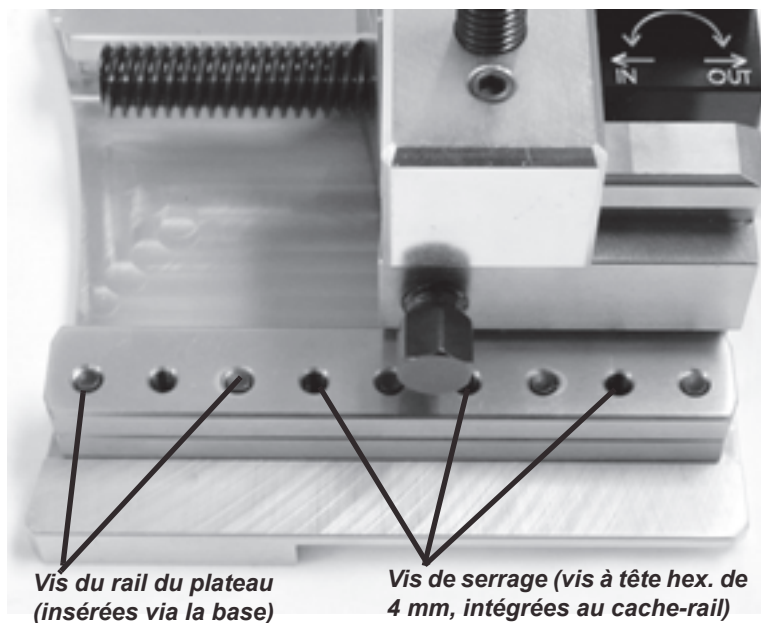
Figure 2-3. Utilisez les vis de serrage sur le rail ajustable pour régler la tension de l'avance sur le plateau. Les vis de serrage alternent avec les vis du rail du plateau.
