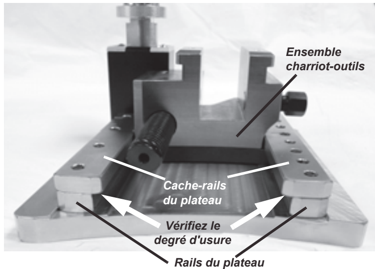
Figure 2-4. L'usure sur la partie inférieure du cache-rails peut donner lieu à un jeu ou à une instabilité du plateau.
